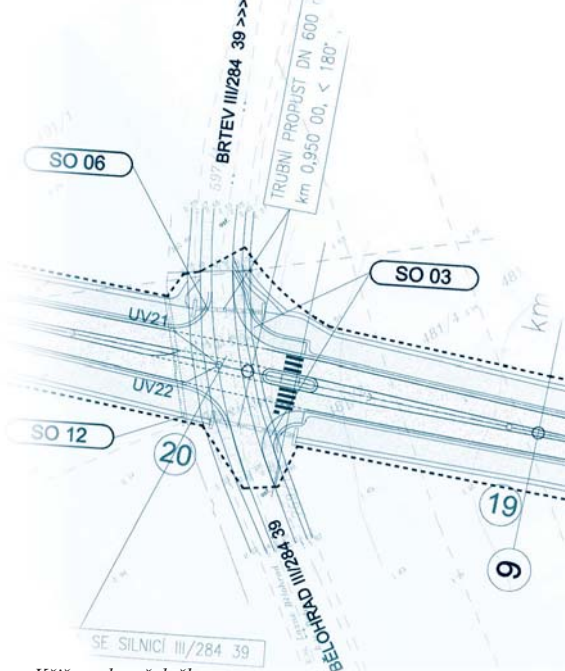
Křížovatka přeložky se silnicí na Brtve
