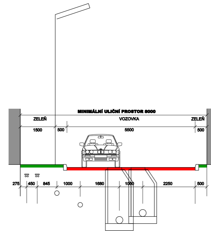
CHARAKTERISTICKÝ PŘÍČNÝ ŘEZ KOMUNIKACÍ 1:100 ULIČNÍ PROFIL "D" OBOUSMĚRNÁ
