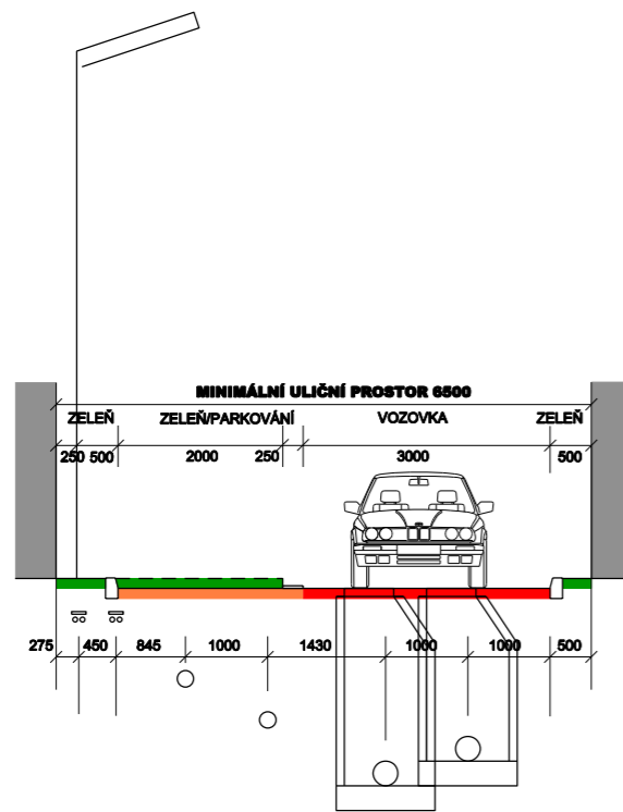
CHARAKTERISTICKÝ PŘÍČNÝ ŘEZ KOMUNIKACÍ 1:100 ULIČNÍ PROFIL "D" JEDNOSMĚRNÁ
